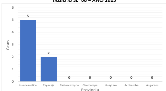
DISTRIBUCION DE EDAS DISENTERICAS POR PROVINCIAS EN MENORES DE 5 AÑOS hasta la SE 06 – AÑO 2025
